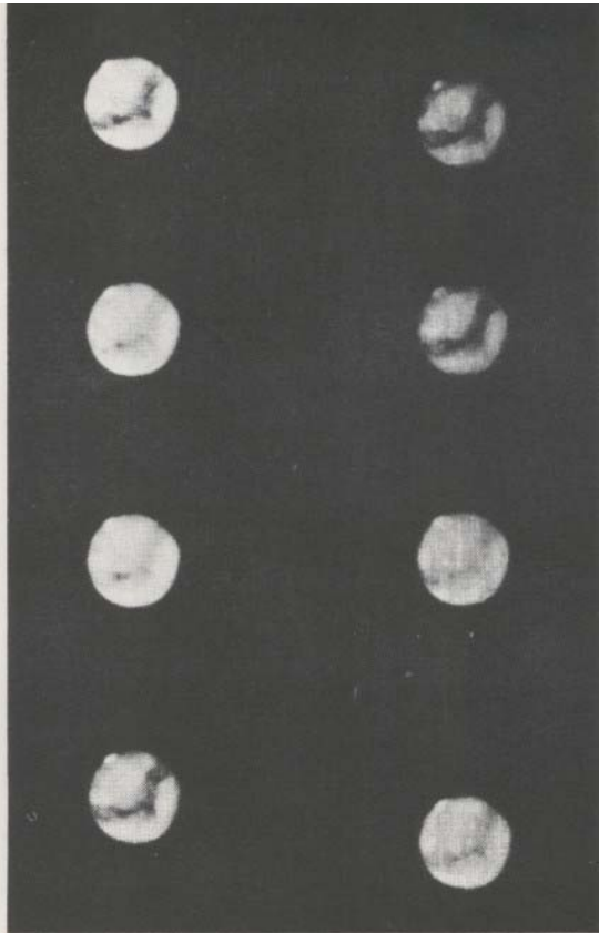
Vues de Mars prises à l'Observatoire de Yerkes le 28 septembre 1902. Elles montrent le cercle blanc, qu'on appelle aussi calotte glacière, se projetant au-delà de la surface de la planète. (D'après l'ouvrage de Marshall B. Gardner.)
