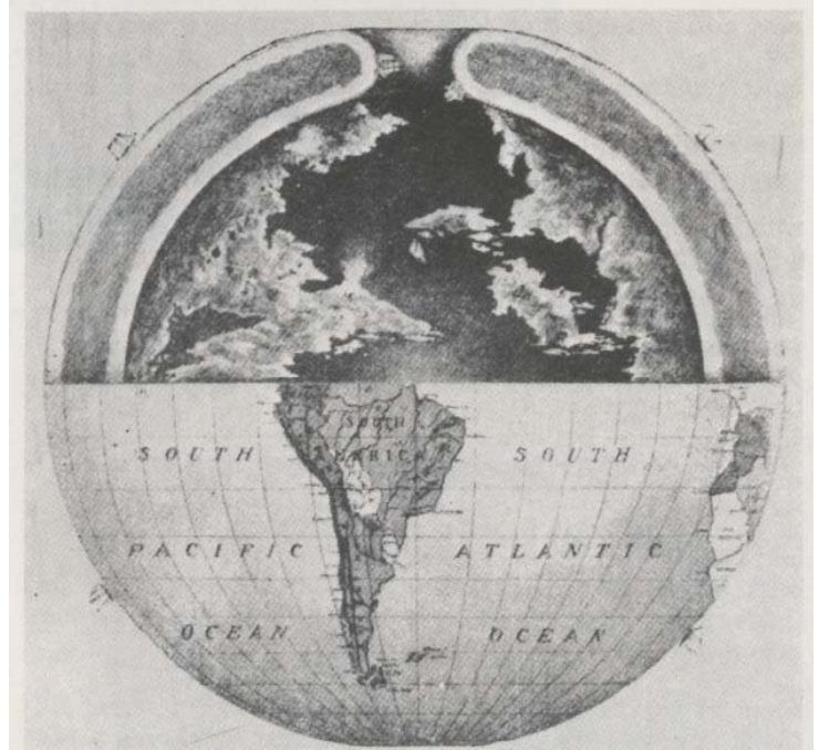
GLOBE MONTRANT UNE SECTION DE L'INTÉRIEUR DE LA TERRE. La Terre est creuse. Les pôles si longtemps cherchés ne sont que des fantômes. Il y a des ouvertures aux extrémités Nord et Sud. A l'intérieur il y a de vastes continents, des océans, des montagnes, des rivières. La vie végétale et animale y est présente. Ce monde est probablement peuplé de races inconnues. (L'auteur, d'après « Fantôme des Pôles », de William Reed, publié par Walter S. Rockey Company, New York, 1906.)
