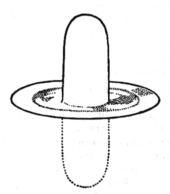
FIGURE. 16. – FORME COMBINÉE DES FORCES
