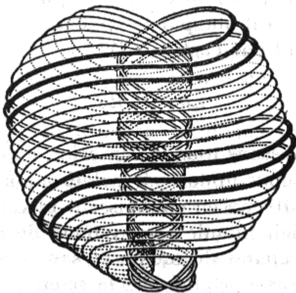
FIGURE. 17. – L'ATOME PHYSIQUE ULTIME
