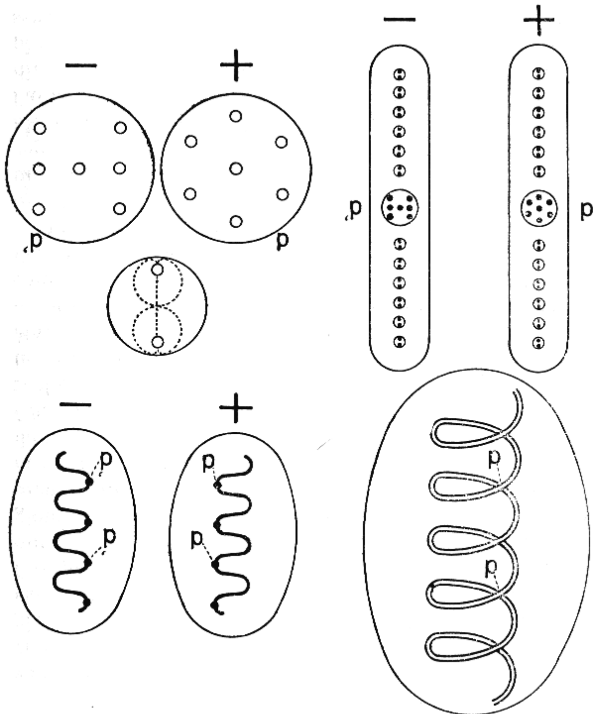
FIGURE. 18. – COMPOSITION DE L'OXYGÈNE
