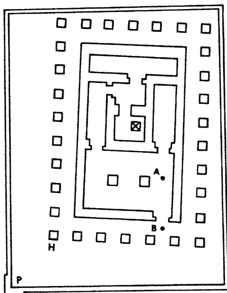
Plan du temple de Satis.
